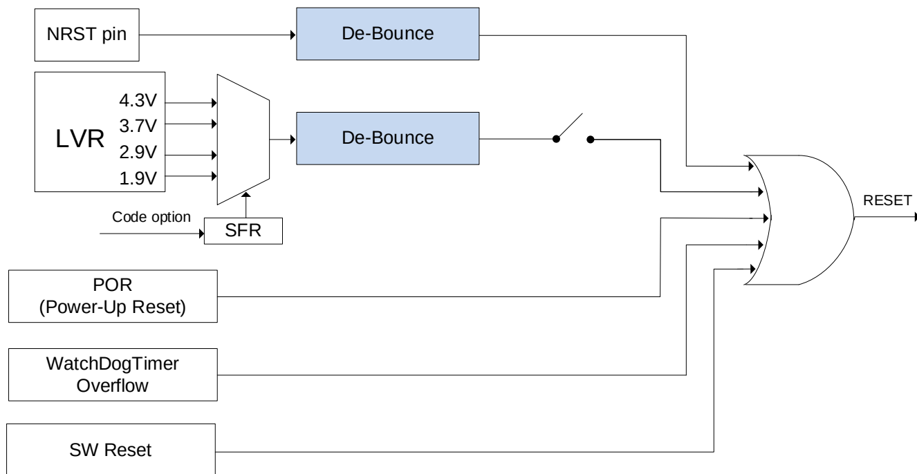
SC32F12T/12G 复位电路图
