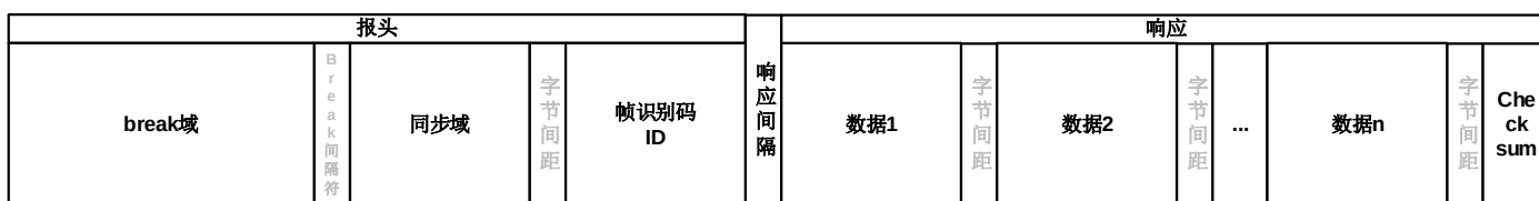
LIN 帧结构图
